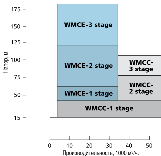
Высоконапорные насосы
