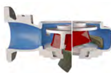
2009 Запуск адаптивного рабочего N-колеса, способного перемещаться вертикально по оси, обеспечивая перекачивание более крупных твердых частиц.
